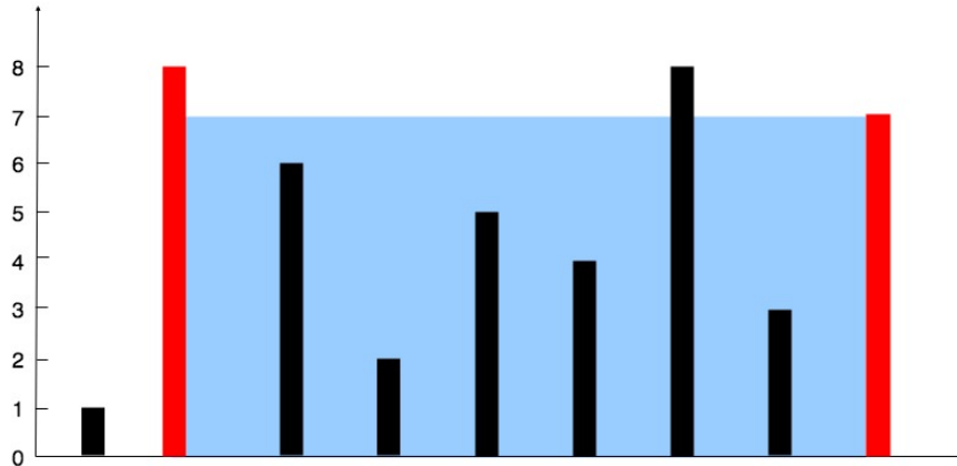
图 2.1. 盛水的容器
