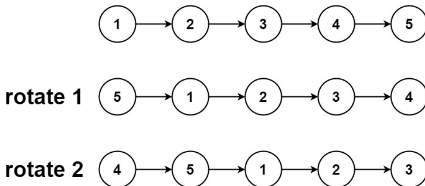
图 1.4. 右移链表
