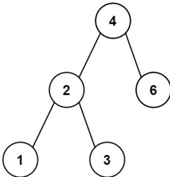
图 13.1. 二叉搜索树
